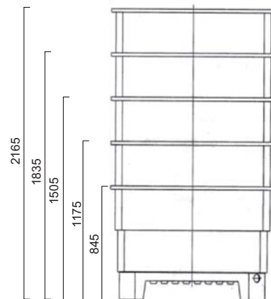
Штабелирование контейнеров КЛ500СП
